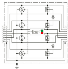
Prinzipschaltbild DPA CL8 EA 4PPOE
